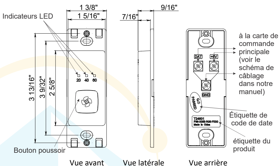
Fig 1.1 données dimensionnelles
