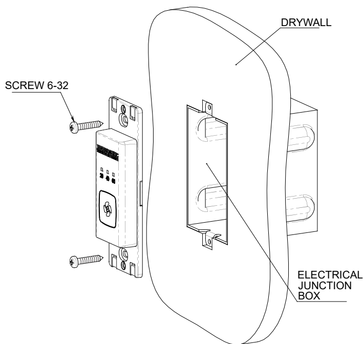
Fig 2.2 Installation avec boîte électrique
